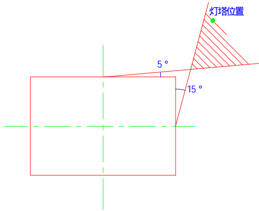
图 10.3.27-1 四塔照明
