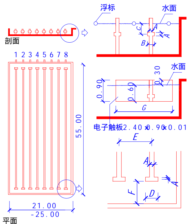
图 7.2.2 标准比赛池平面、剖面
